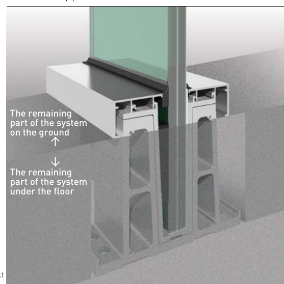
In floor installation detail Detailansicht: Montage im Boden versenkt Details d'application dans le sol
