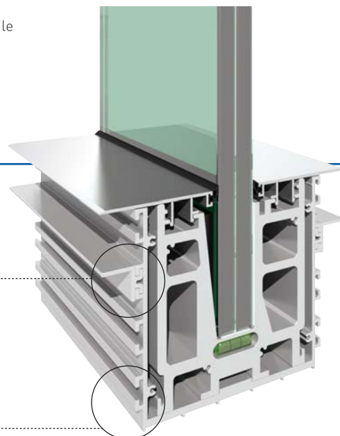
Height Adjusting U Case Profile Option Höheneinstellungsprofil für U Gehäuse Option pour cadre réglable
