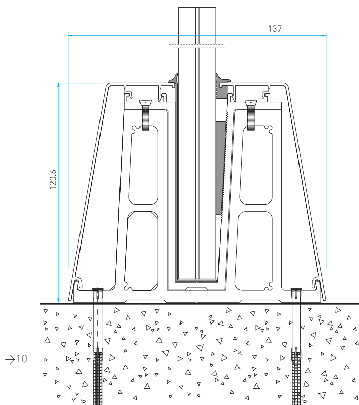
View of in floor detail Detailansicht: Montage im Boden versenkt Vue sur le sol en détail
